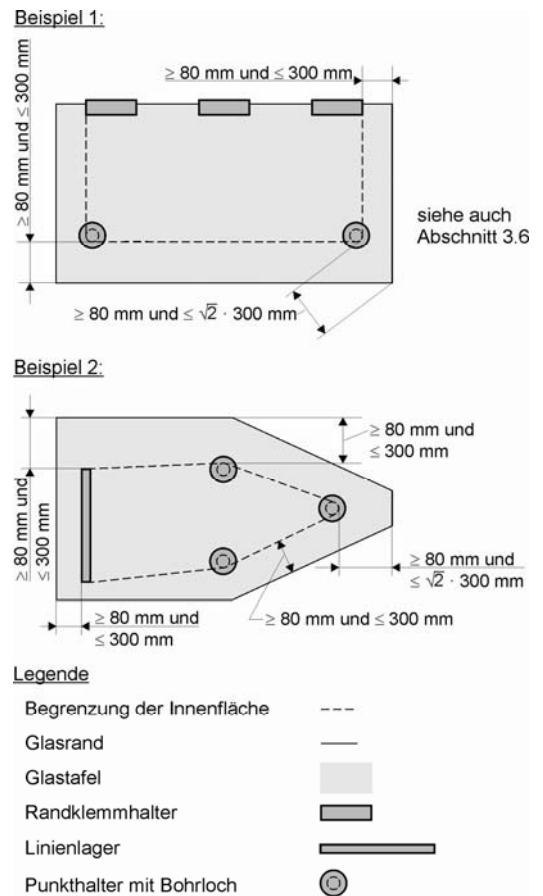
Bild 1: Prinzipskizze Glasauskragung
