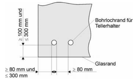
Bild 2: Randabstände Bohrloch
